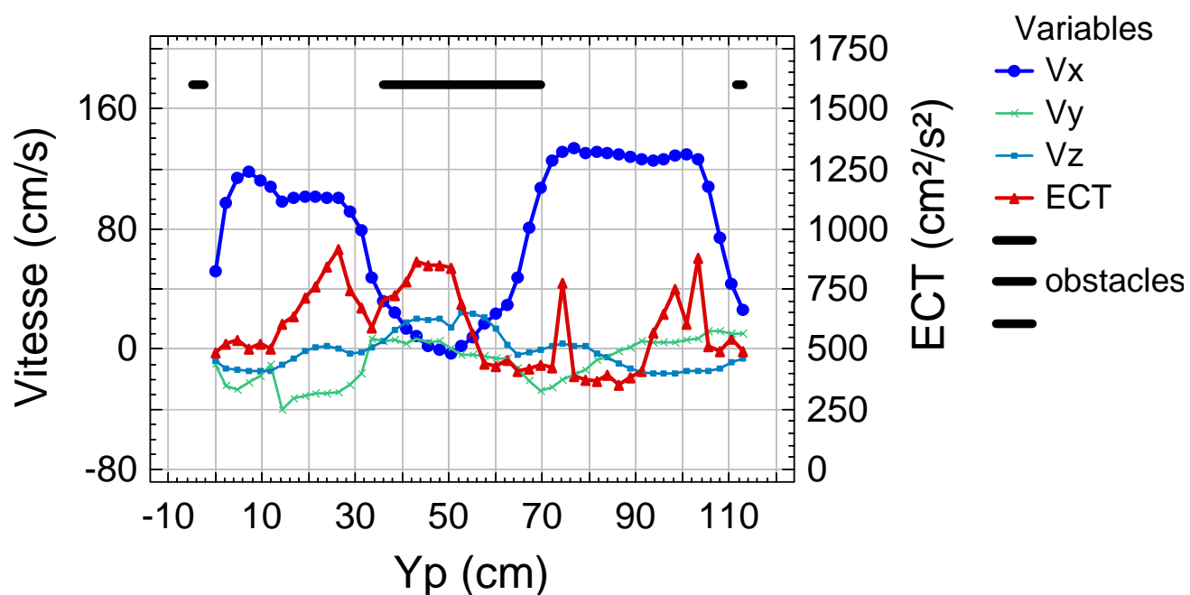
Figure 9. Profils des vitesses et de l'Énergie Cinétique Turbulente (en \text{cm}^2/\text{s}^2 ) Pente 5% - filtre GN+1.5g – transect 24 cm
