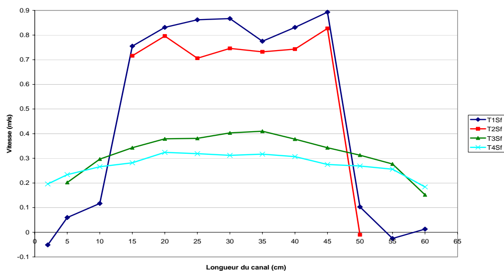
Figure 42. Profils des vitesses à la sortie du canal
