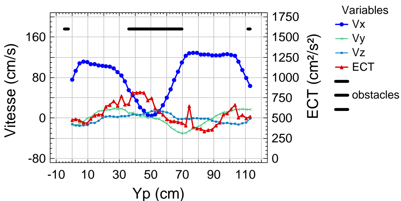
Figure 10. Profils des vitesses et de l'Énergie Cinétique Turbulente (en \text{cm}^2/\text{s}^2 ) Pente 5% - filtre GN+1.5g – transect 36 cm
