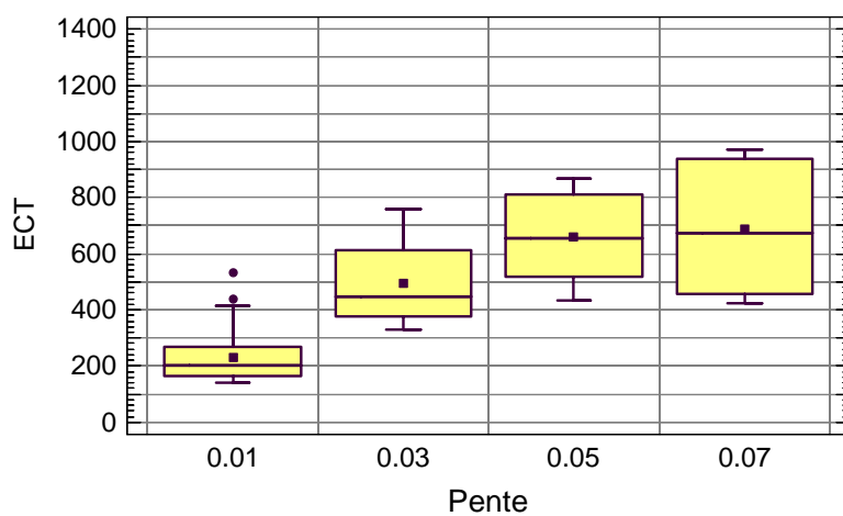
Figure 22. Boîtes à moustache de l'ECT (en \text{cm}^2/\text{s}^2 ) en fonction de la pente ( V_m < 30 cm/s)
