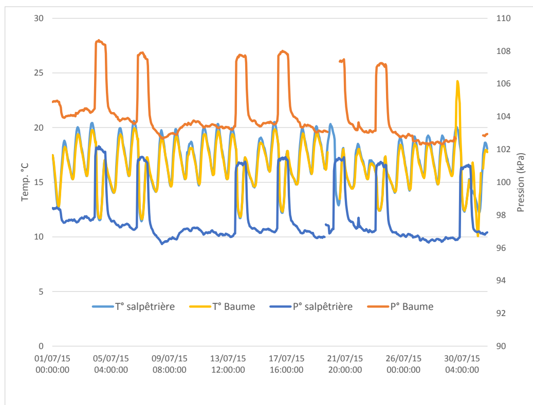
Figure 13 : Evolution des pressions (proxy du débit) et températures de l'eau enregistrées sur les deux stations au mois de juillet 2015 (les valeurs brutes de pression diffèrent car la profondeur de pose est différente entre les deux stations)
