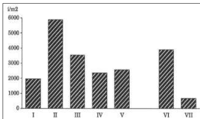
Figure 22 : Evolution amont - aval des densités totales en invertébrés sur la Moyen Verdon (Galvin, 1989) (I = Castellane ; II = Pont de Taloire ; III = Pont de Soleils ; IV = Pont de Carajuan ; V = couloir Samson ; VI = Baou ; VII = Jabron)
