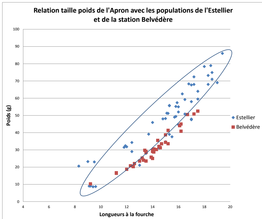
Fig. 4. Courbes taille/poids des aprons capturés sur le Verdon en 2012, sexes confondus.
