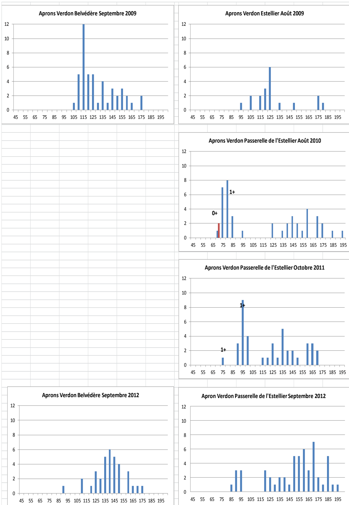
Fig.3. Histogrammes de captures d'aprons sur les deux stations entre 2009 et 2012, la barre rouge en août 2010 indique un individu 0+.
