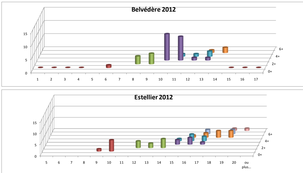
Fig. 8. Distribution en taille des individus pour les différentes classes d'âge.
