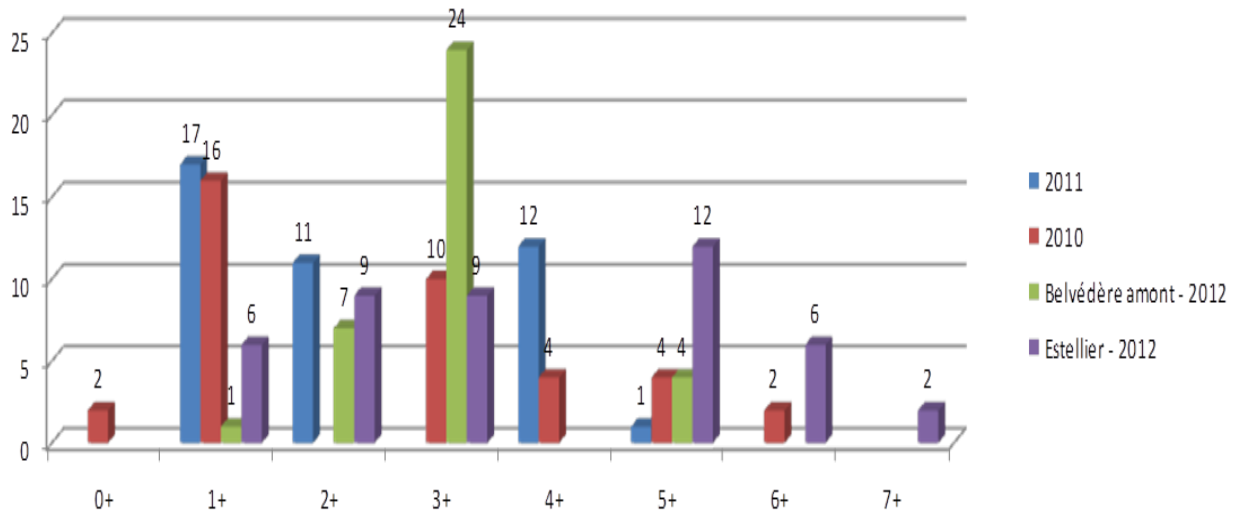
Fig. 7. Distribution des individus capturés en 2010 et 2011 dans les différentes classes d'âge, 41 individus en 2011 et 38 individus en 2010 ont pu faire l'objet de l'analyse.
