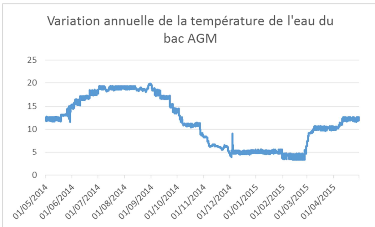
Figure 26 : cycle thermique du bac AGM
