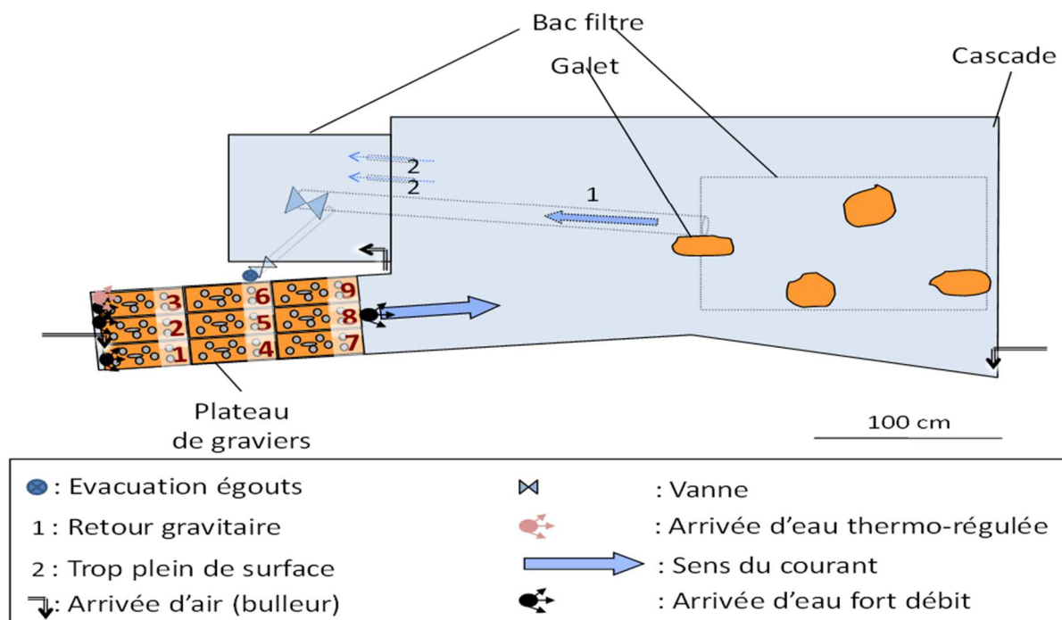
Figure 4 : vue de dessus de bac AGM
