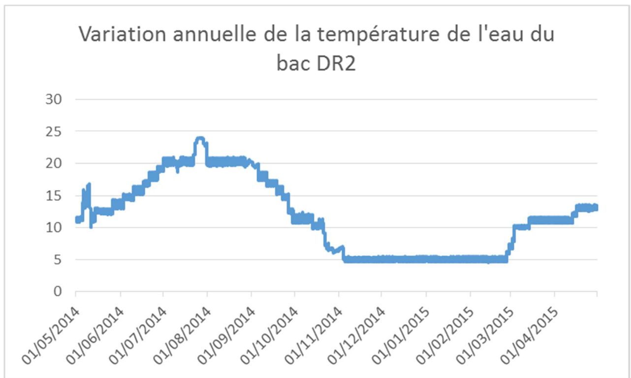
Figure 25 : cycle thermique du bac DR2
